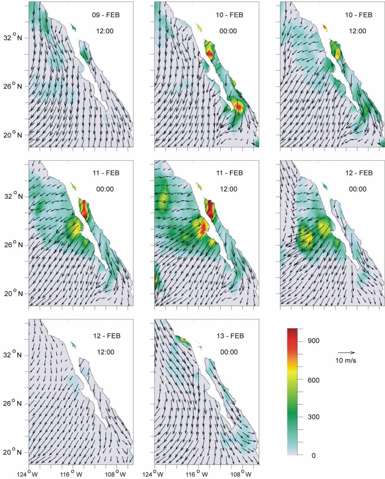
Figura 3a–h. Vectores de velocidad del viento superficial del 9 al 13 de febrero de 2002. Los contornos de color indican el índice de variación ( \text{m}^3/\text{s}^3 ). La fecha y la hora se indican con respecto al meridiano de Greenwich.
