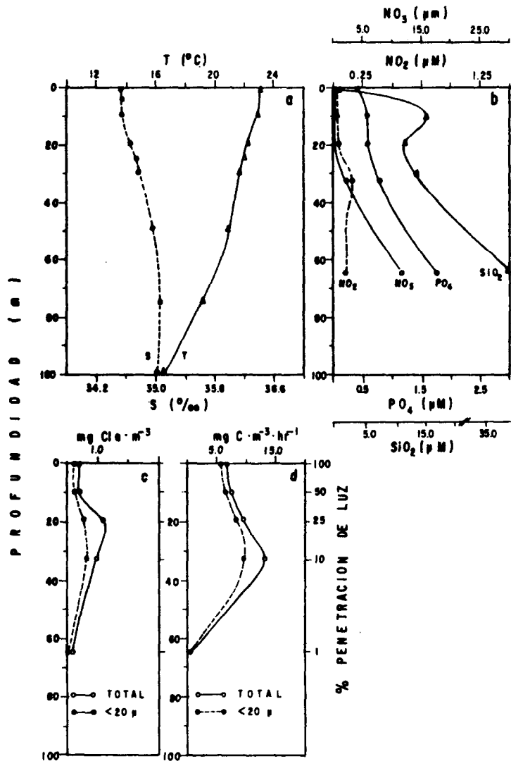
Figura 2. Perfiles verticales de: a) temperatura ( T^{\circ}\text{C} ) y salinidad ( S^{\circ}/\text{oo} ); b) nitratos, nitritos, fosfatos y silicatos ( \mu\text{M} ); c) clorofila a total y para la fracción del nanofitoplancton ( \text{mg Chl a m}^{-3} ); d) productividad primaria total y para la fracción del nanofitoplancton ( \text{mg C m}^{-3}\cdot\text{h}^{-1} ), para la estación nueve en marzo 1983.
