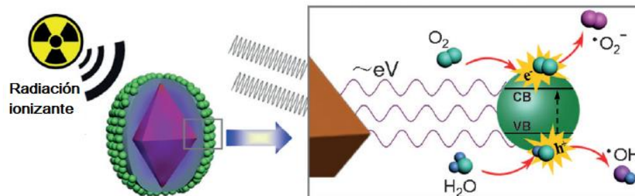
Figura 15. Los pares electrón–hueco ( e^- - h^+ ) se forman después de la exposición a la radiación ionizante.
