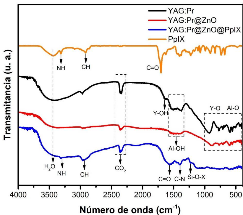
Figura 24. Espectros de infrarrojo de YAG:Pr (línea negra), YAG:Pr@ZnO (línea roja), YAG:Pr@ZnO@PpIX (línea azul) y PpIX (línea amarilla).
