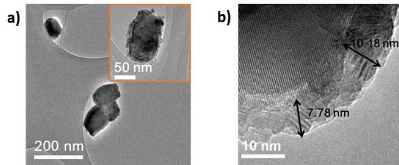
Figura 21. Imágenes obtenidas por TEM de YAG:Pr@ZnO a a) baja y b) alta ampliación.
