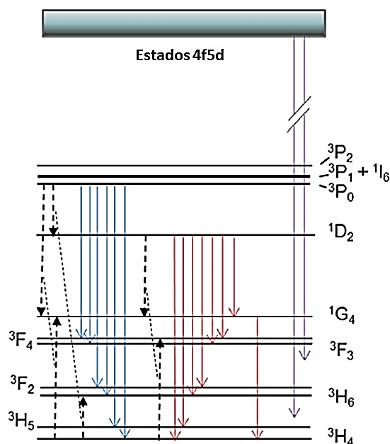
Figura 3. Esquema de los niveles de energía y procesos de relajación de YAG:Pr (Cavalli et al., 2015).
